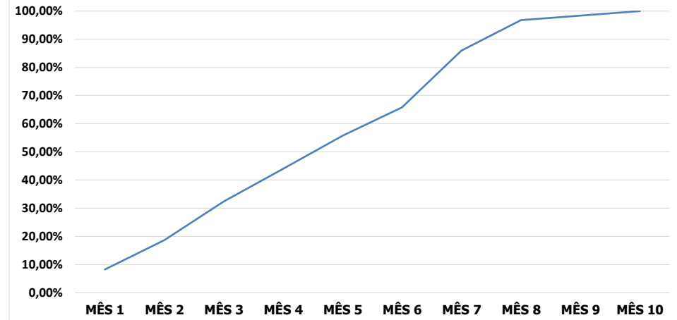
CURVA S - SERVIÇOS CUMULADOS
